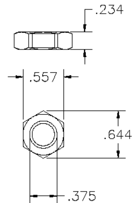
P/N 1000764 3/8 Jam Nut
