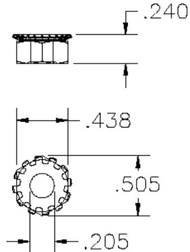
P/N 1000768 1/4 Kep Nut
