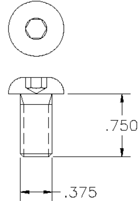
P/N 1008540 MS 3/8 x 3/4 sckt btn hd
