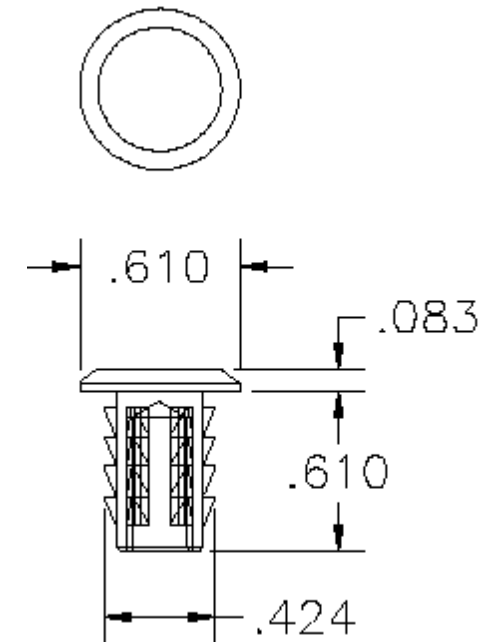
P/N 2043272 1/4 insert Nut
