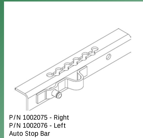
P/N 1002075 - Right P/N 1002076 - Left Auto Stop Bar
